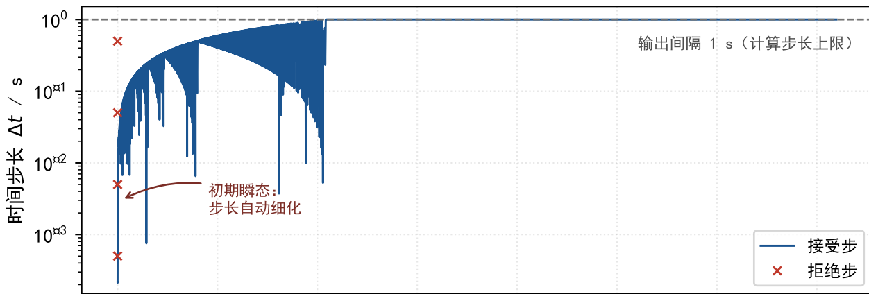
(a) 自适应时间步长历史：输出每 1 s 精确落点，计算步长由误差控制独立决定
