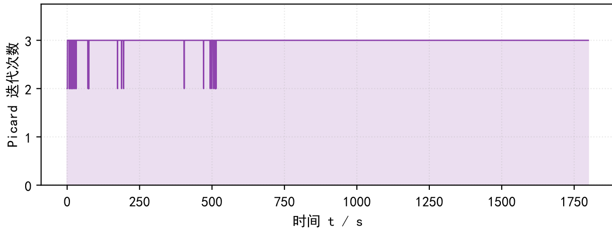
(b) 每步 Picard 迭代次数 (尖峰对应含水率陡变、 D(C) 刚性段)
